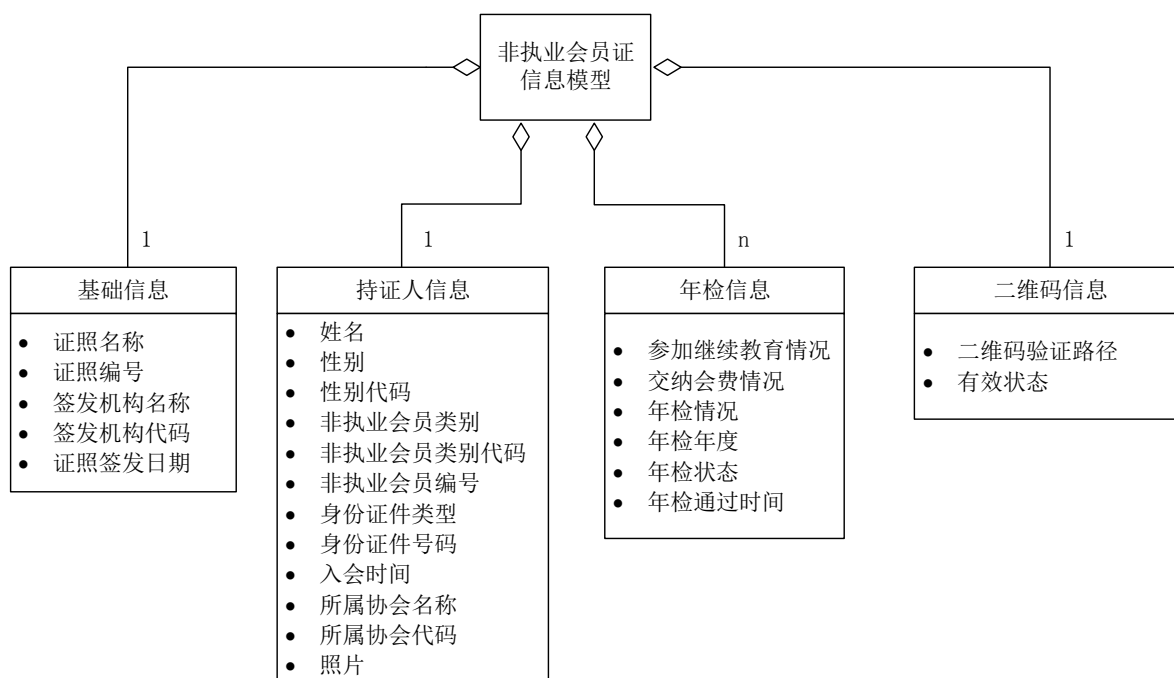
图1 非执业会员证电子证照信息模型 UML 类图
