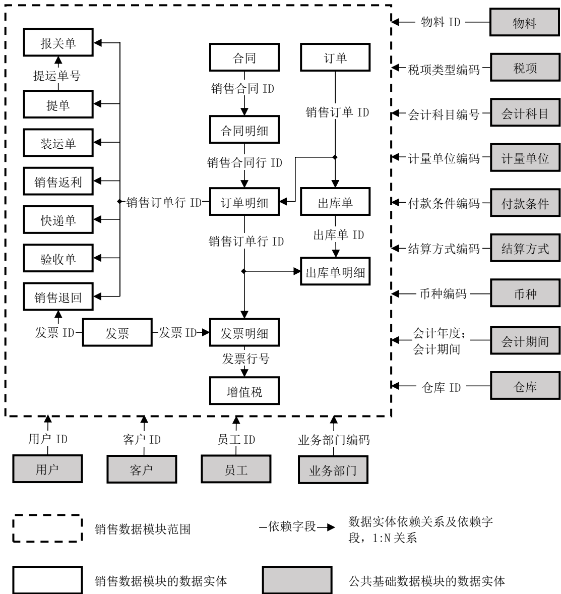
图 1 销售数据实体关系图
