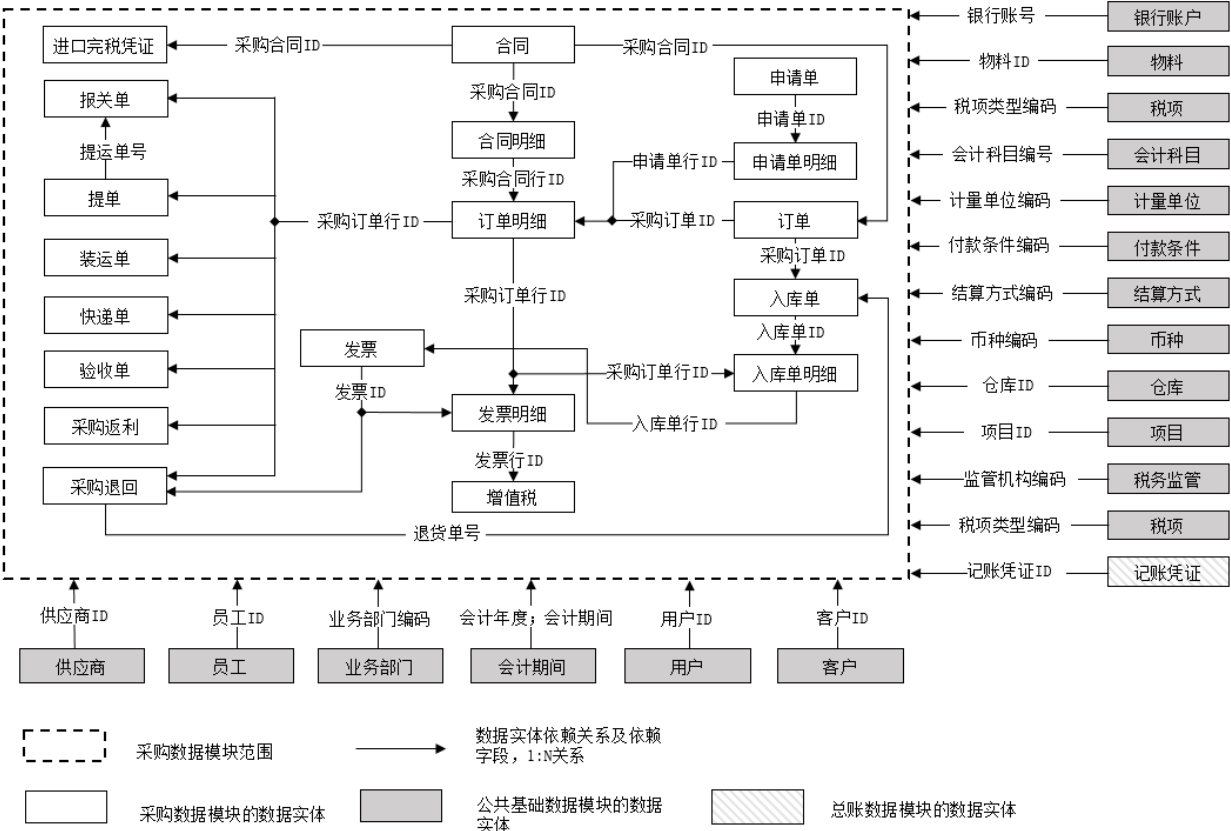
图1 采购数据实体关系图
