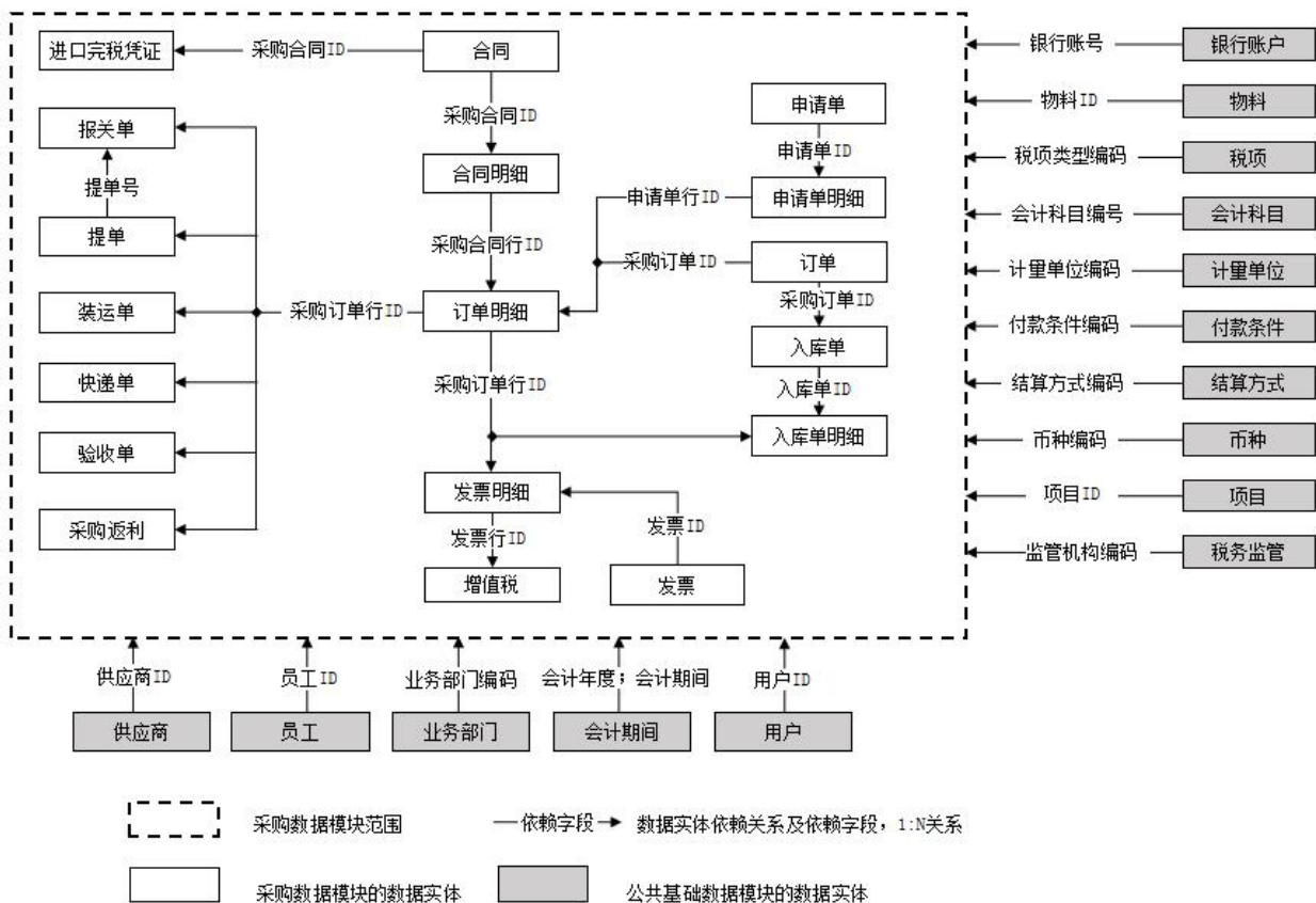
图 1 采购数据实体关系
