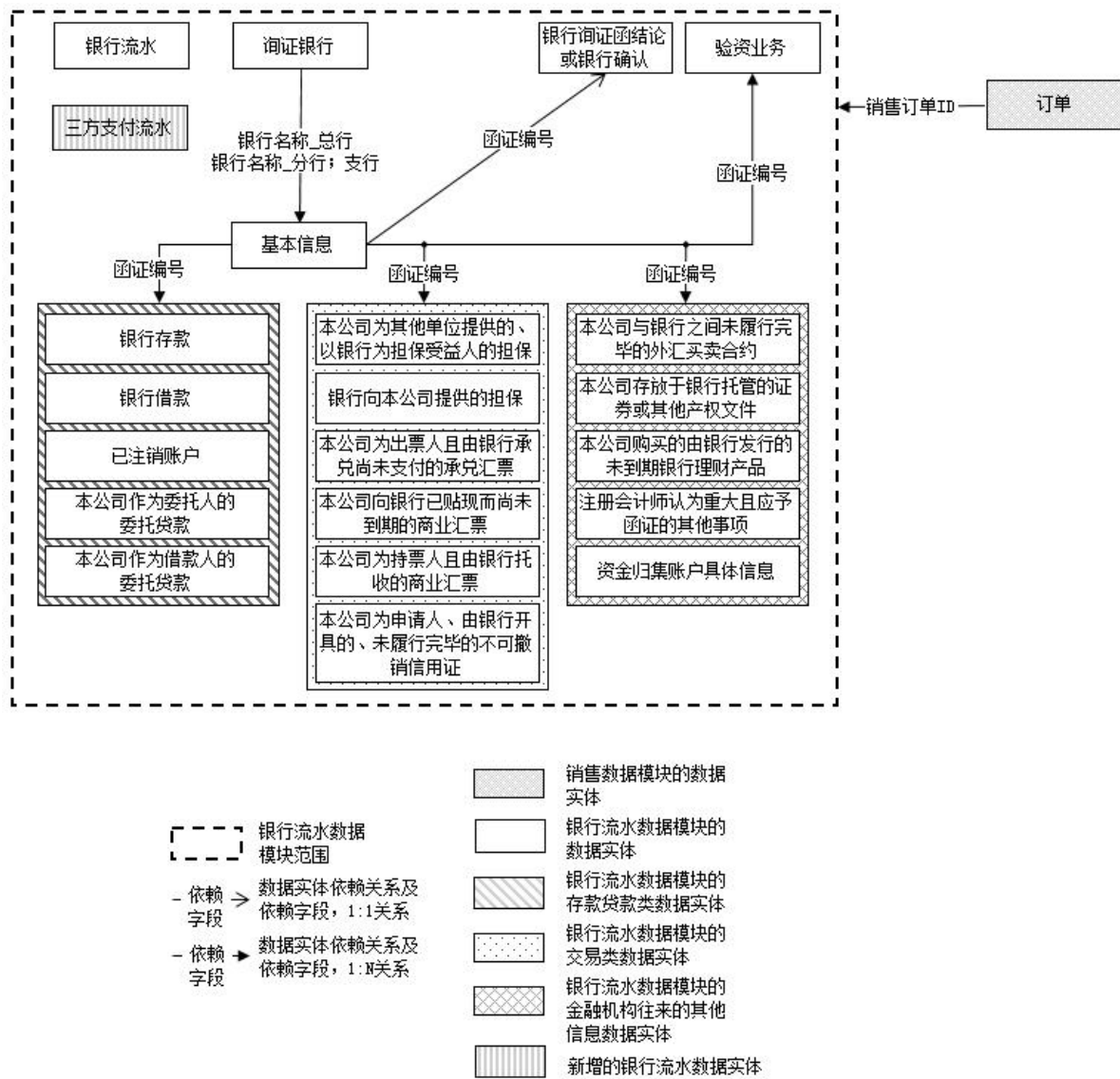
图4 银行流水数据实体关系
