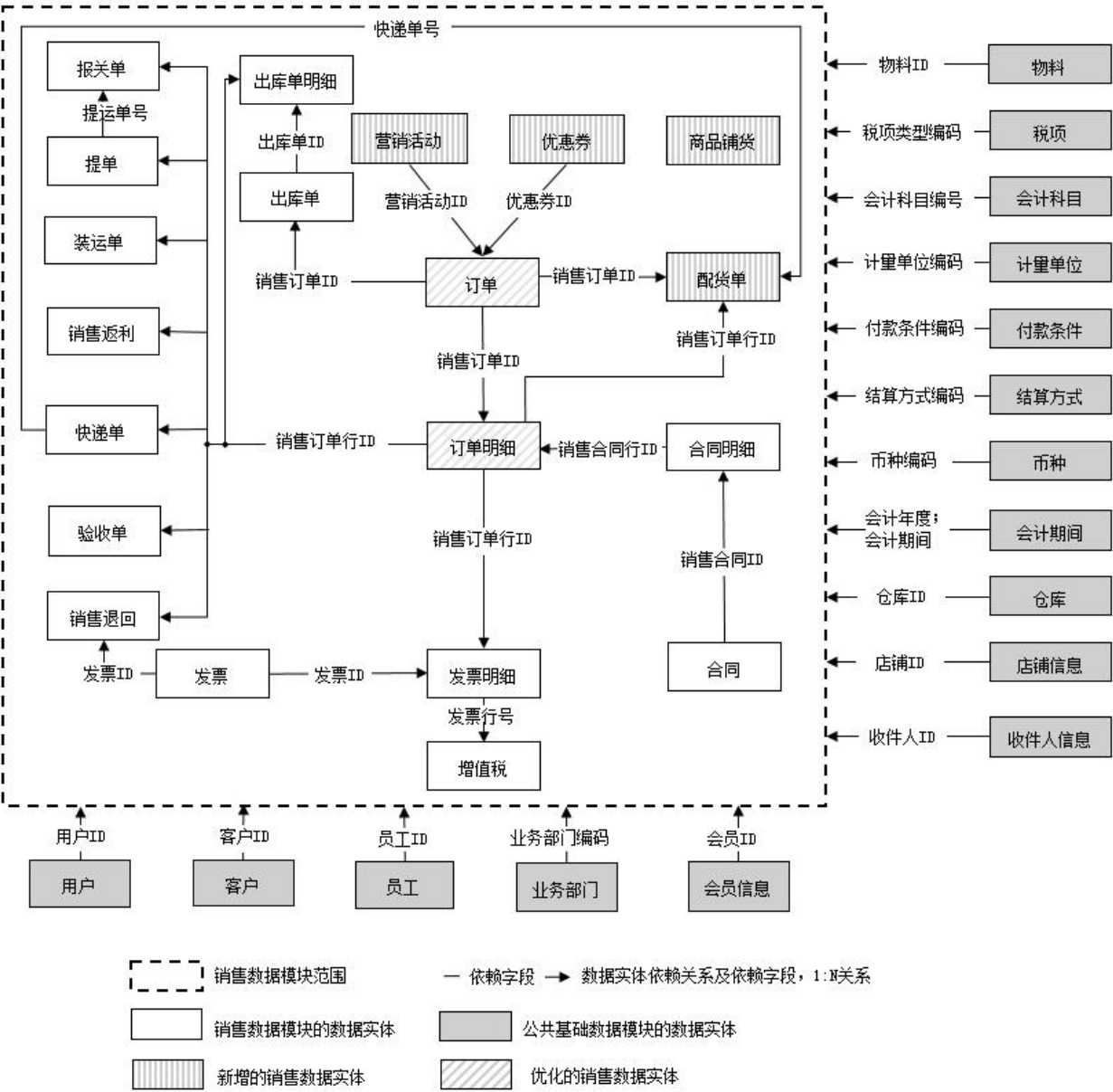
图3 销售数据实体关系
