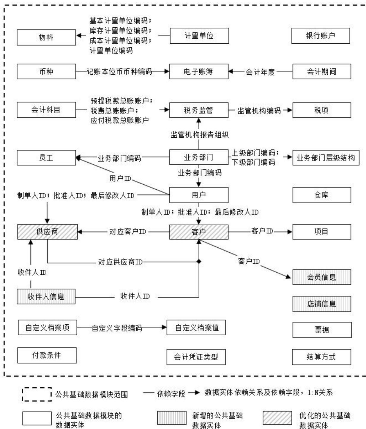
图2 公共基础数据实体关系
